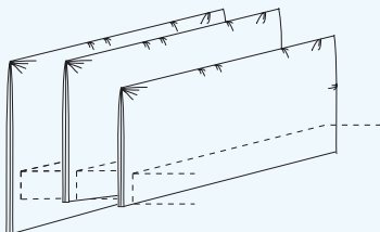
SLIM schwebend Höhe: 74/94/114 cm, Tiefe: 5 cm SLIM aufstehend Höhe: 94/114 cm + 2 cm Bodenleiste Tiefe: 5 cm Breite: 128-228 cm
