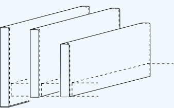
BOHEMIAN A schwebend Höhe: 94/114 cm, Tiefe: 10 cm BOHEMIAN A aufstehend Höhe: 125 cm + 2 cm Bodenleiste Tiefe: 10 cm, Breite: 122-222 cm
