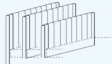
BOHEMIAN F schwebend Höhe: 94/114 cm, Tiefe: 8 cm BOHEMIAN F aufstehend Höhe: 125 cm + 2 cm Bodenleiste Tiefe: 8 cm, Breite 122-222 cm
