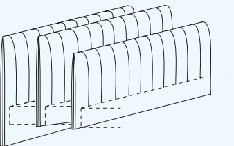
SLIM QUILT schwebend Höhe: 74/94/114 cm, Tiefe: 8 cm SLIM QUILT aufstehend Höhe: 94/114 cm + 2 cm Bodenleiste Tiefe: 8 cm, Breite: 128-228 cm
