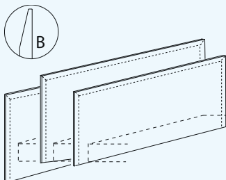
SMART B schwebend, 3-seitig nach hinten abgeschrägt Höhe: 74/94 cm, Tiefe: 3 cm SMART B aufstehend, 3-seitig nach hinten abgeschrägt Höhe: 94 cm Tiefe: 3 cm, Breite 122-222 cm
