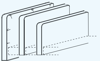
BOHEMIAN D schwebend mit Paspel Höhe: 94/114 cm, Tiefe: 12 cm BOHEMIAN D aufstehend Höhe: 125 cm + 2 cm Bodenleiste Tiefe: 12 cm, Breite 122-222 cm
